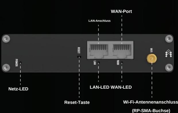
VORDERANSICHT
